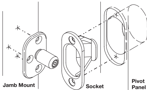
Socket
